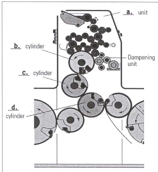
常見之張頁式平版印刷單元
